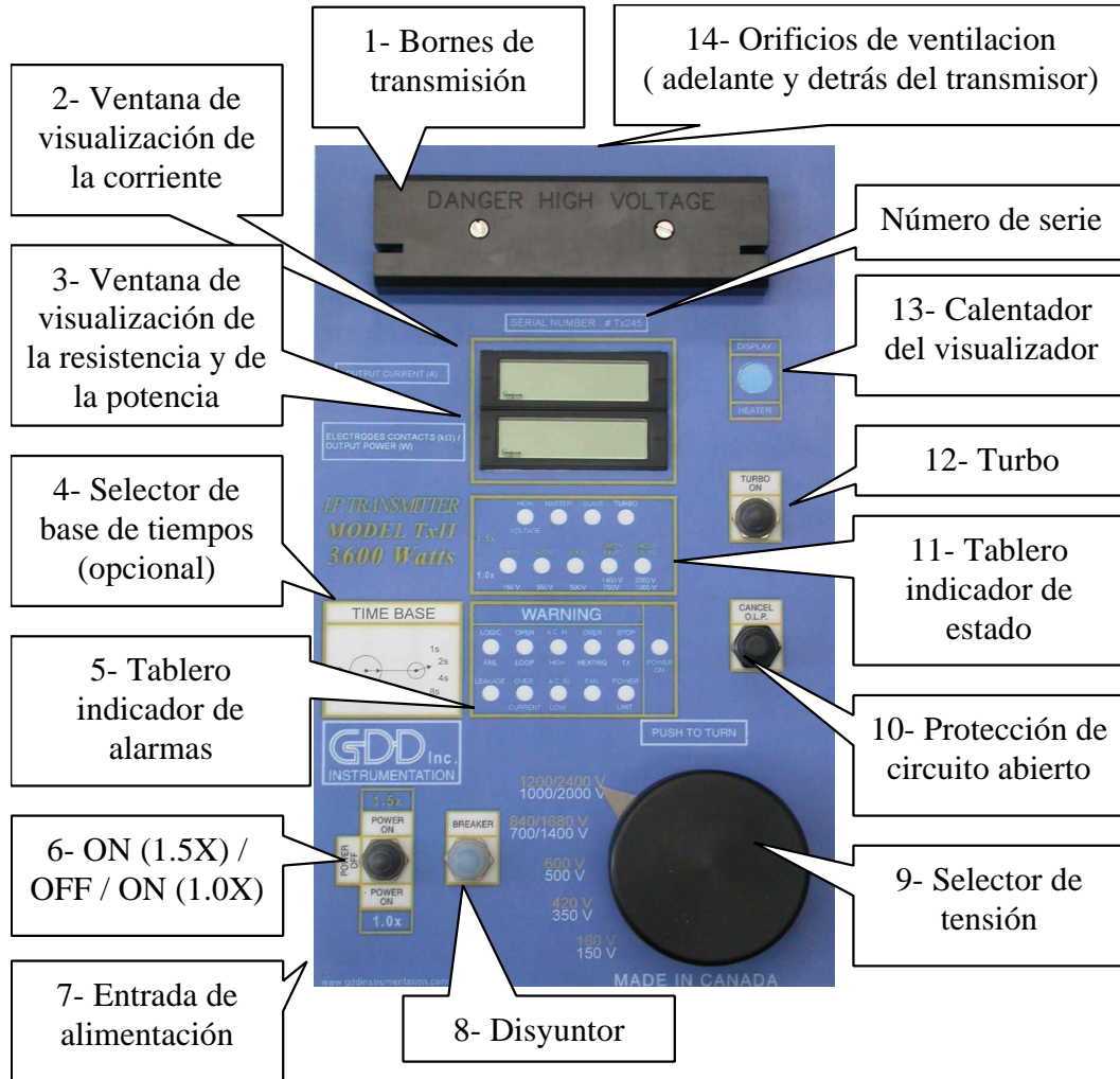
Figura 1: Componentes del transmisor
